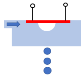
Thermal inkjet
